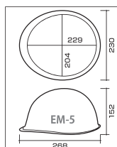
EM-5型寸法図
