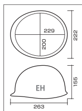
EH型寸法図
