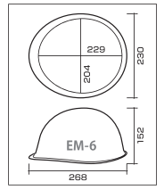
EM-6型寸法図
