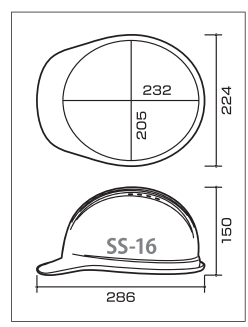
SS-16V型寸法図
