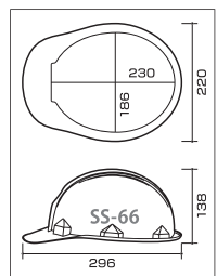
SS-66型寸法図
