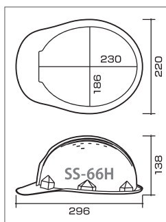
SS-66H型寸法図
