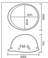
FM-6型寸法図
