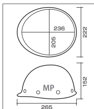
MP型寸法図
