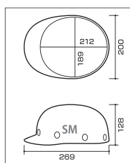
SM型寸法図
