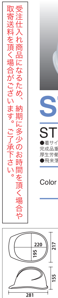
ST#121-CZ型寸法図
