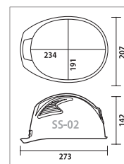
SS-02型寸法図
