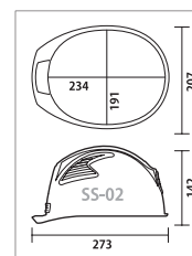
SS-02型寸法図
