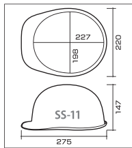
SS-11型寸法図
