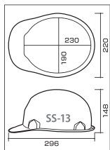
SS-13型寸法図
