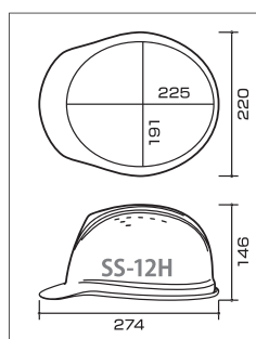
SS-12H型寸法図
