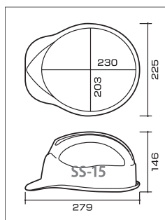
SS-15型寸法図
