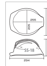
SS-18V型寸法図
