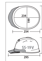
SS-19V型寸法図
