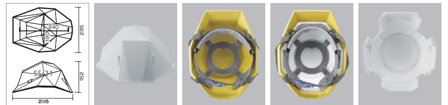
SS-21型 寸法図
