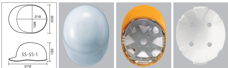
SS-55-1型寸法図
