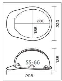
SS-66型寸法図
