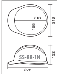
SS-88-1N型寸法図
