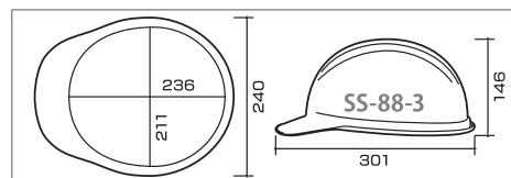
SS-88-3型寸法図
