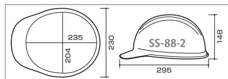
SS-88-2型寸法図
