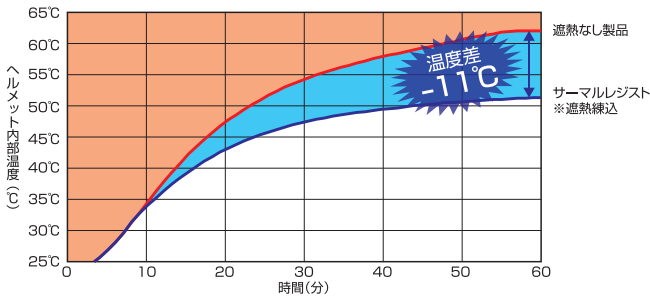
遮熱性能比較実験(当社試験)
