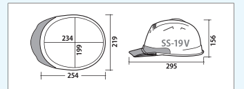
SS-19V型寸法図
